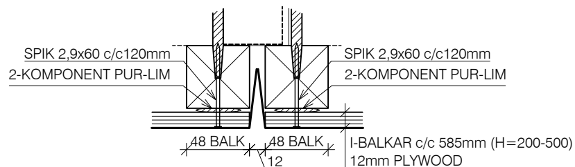
DETALJ B, SKALA 1:4
