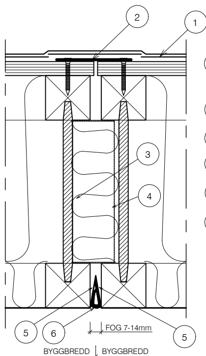
DETALJ A -1:4
